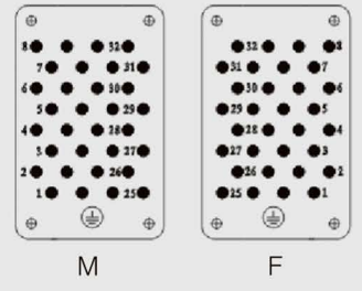
接插针排序
